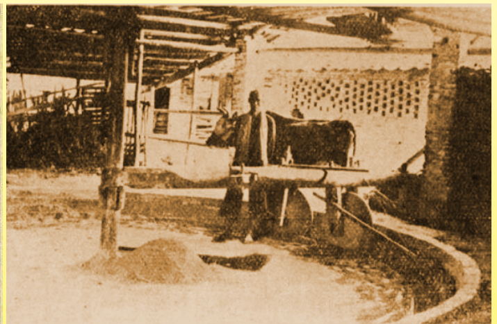
Molienda de caolín en un molino accionado por un buey (1939, Vietnam, Boletín Económico de la Indochina)
