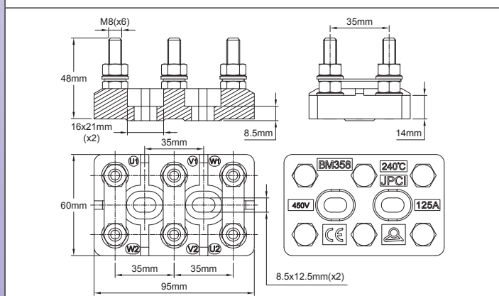
Modelo 125A 450V (espaciado de terminales 35 mm con tornillos M8)
