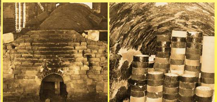
Dragón chino tradicional horno (龙窑 Long Yao). Boca de alimentación y procedimiento de llenado de porcelana eléctrica (colección privada)
