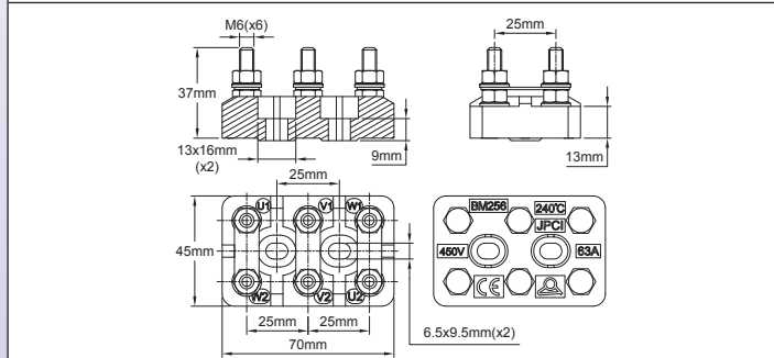
Modelo 63A 450V (espaciado de terminales 25 mm con tornillos M6)
