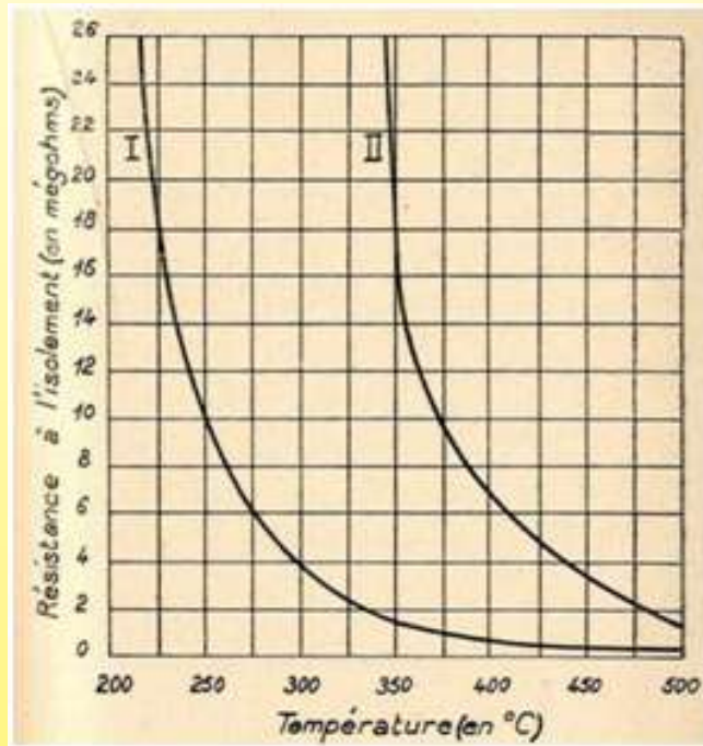
Variaciones de la resistencia de aislamiento entre la porcelana (I) y la esteatita (II), medidas en muestras idénticas en 1945 (Matériaux électrotechniques modernes de 1945, museo Ultimheat)
