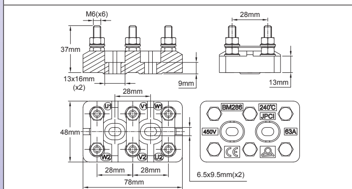
Modelo 63A 450V (espaciado de terminales 28 mm con tornillos M6)
