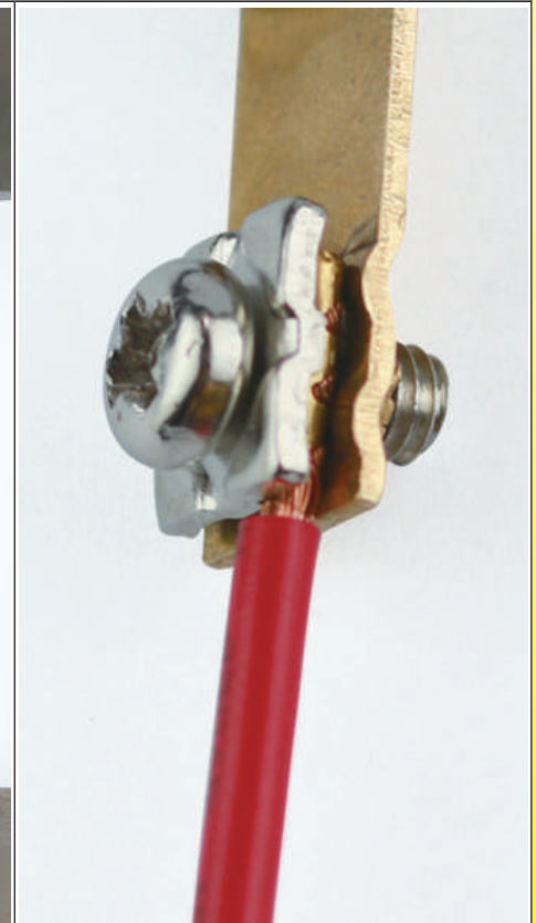
Detalle del terminal
