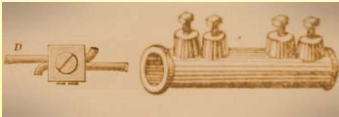
Terminales de tornillo de 1892 (Manuel pratique de l'installation de la lumière électrique. Installations privées, de J.-P. Anney)
