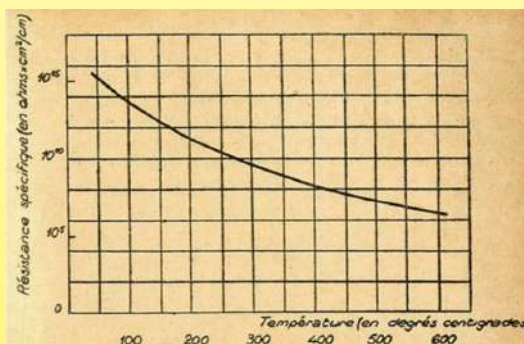
Variación de la resistencia de la porcelana en función de la temperatura indicada en ohmios.cm/cm 2 (curva logarítmica). Cuando la temperatura es de entre 20 °C y 300 °C, su resistencia se divide entre 10.000 (Matériaux electrotechniques modernes de 1945, museo Ultimheat)
